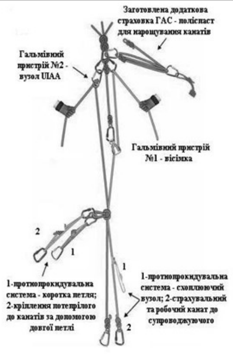
Рисунок. 8.2 – Кріплення потерпілого та супроводжувача до спускових мотузок та систему для сидіння потерпілого
