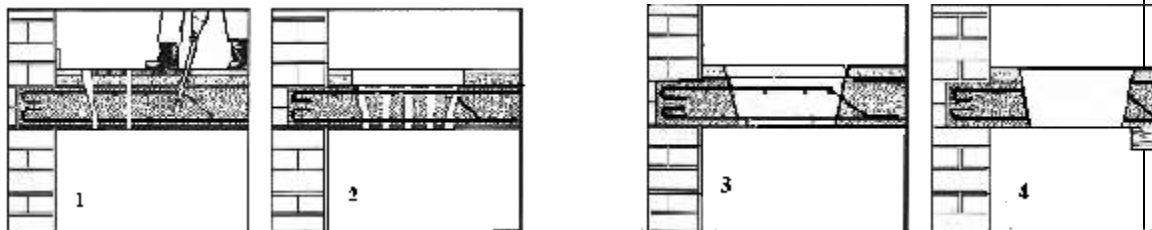
Рис. 6.25. Порядок виготовлення пролому стелі
