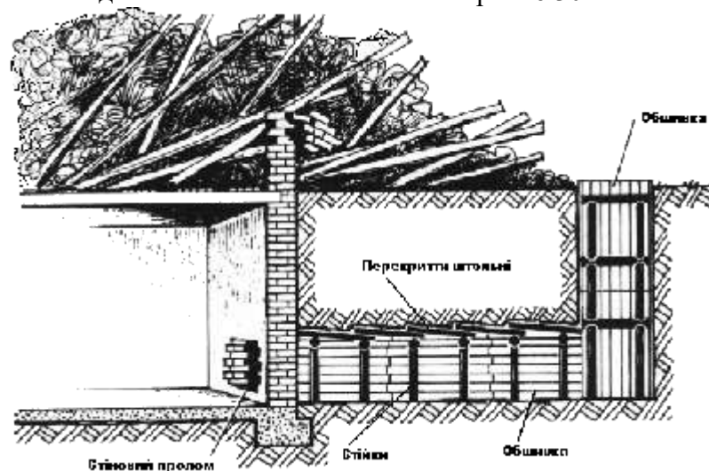
Рис. 6.30. Шахта і штольня
