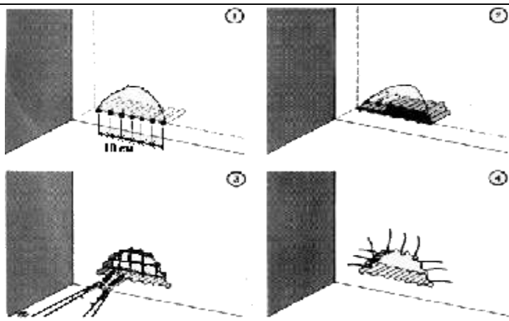
Рис. 6.23. Порядок виконання стінового пролому а-В цегляній стіні. б-В бетонній стіні
