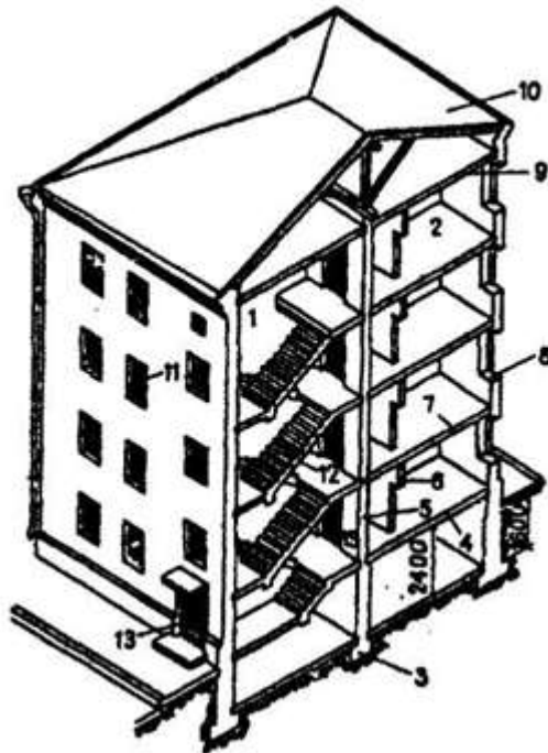
Рис. 2.1. Об'ємно-планувальні та конструктивні елементи будинку
